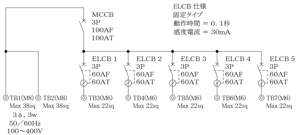
結線図
