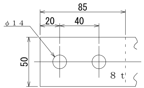
入力端子詳細図 Input Terminal detail drawing
