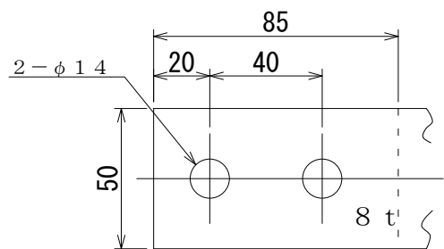
入力端子詳細図 Input Terminal detail drawing
