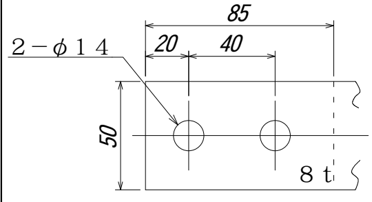
入力端子詳細図 Input Terminal detail drawing
