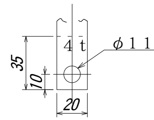
出力端子詳細図 Output Terminal detail drawing
