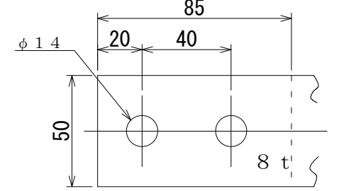
入力端子詳細図 Input Terminal detail drawing
