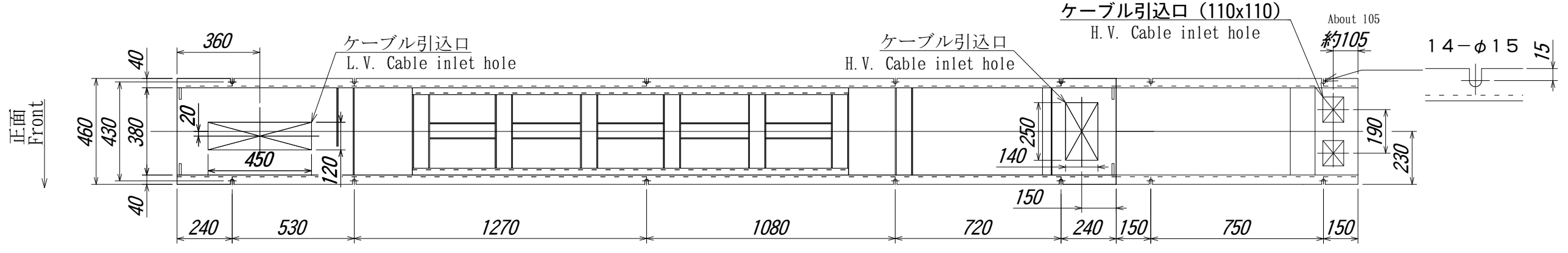
ケース上部から見たベース詳細図 Base detail drawing from the case upper side
