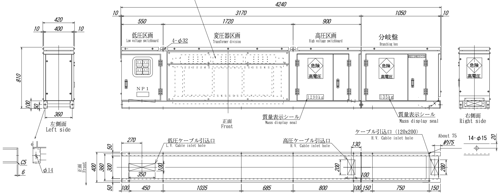
ケース上部から見たベース詳細図 Base detail drawing from the case upper side
