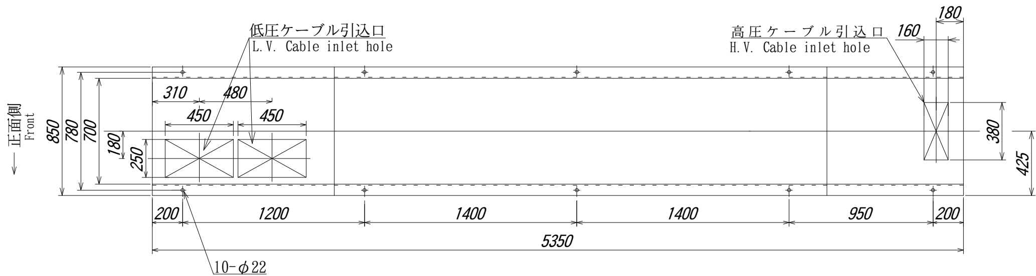
(ケース上面から見たベース詳細図) Base detail drawing from the case upper side
