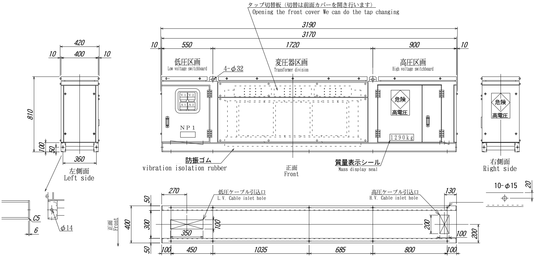
ケース上部から見たベース詳細図 Base detail drawing from the case upper side
