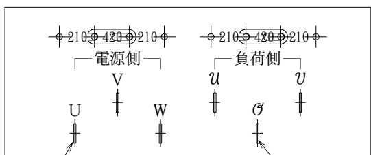
1次端子 端子板 2次端子
